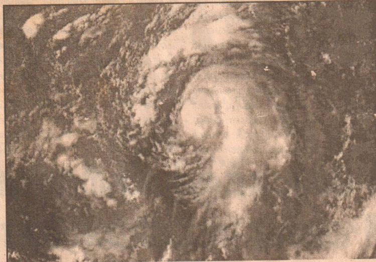
வடகரோலீனா கரையோரப் பகுதியில் நேற்று முன்தினம் மையம் கொண்டிருந்த "அலைக்ஸ்" என்ற புயலின் செய்மதிப் படம்.
